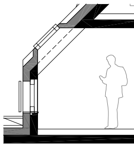
SCHNITT 1-1
