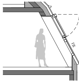
SCHNITT A
